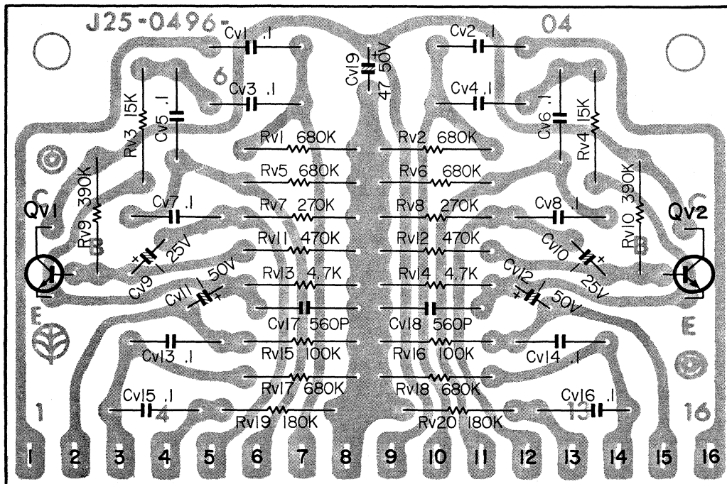
QV1,2 2SC871
