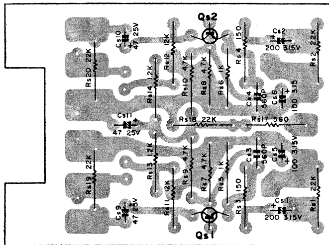
Qs1,2 2SC458LG(B)
